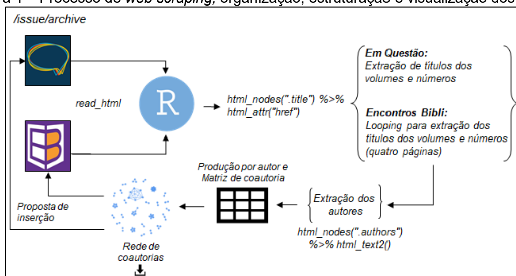
Figura 1 – Processo de web scraping , organização, estruturação e visualização dos dados
