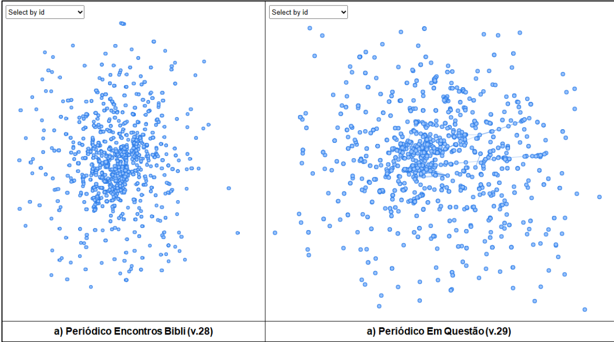
Figura 5 - redes de coautorias de ambas revistas contendo todos autores para ambas revistas com frequência mínima de coautoria entre autores igual a 1
