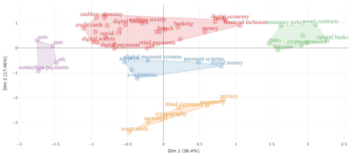
Figura 10 - Análise fatorial
