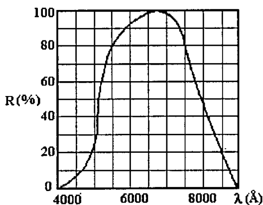
Fig. 2: Sensibilidade de um LDR para vários comprimentos de onda da luz incidente ( \lambda ).
