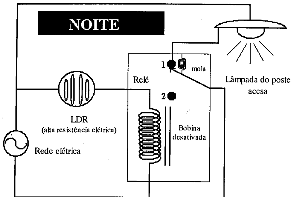
Fig. 3b: À noite, a resistência elétrica do LDR é alta pois a luz solar não está presente, impedindo que a corrente elétrica atravessasse a bobina, que deixa de atuar como ímã. A mola obriga então a chave do relé a retornar para a posição 1, acionando a lâmpada, que se apagará automaticamente no dia seguinte, uma vez que o circuito volta à situação mostrada na Fig. 3 a.
