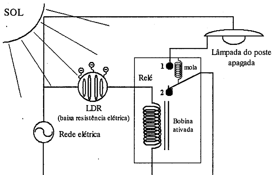
Fig. 3a: Durante o dia a luz solar promove no LDR elétrons ligados a elétrons livres, conforme indicado acima. A resistência elétrica do LDR se torna mais baixa e a corrente elétrica atravessa a bobina, gerando um campo magnético, como se ela fosse um ímã. A chave do relé é então atraída para a posição 2, impedindo que a corrente elétrica passe pelo filamento da lâmpada.
