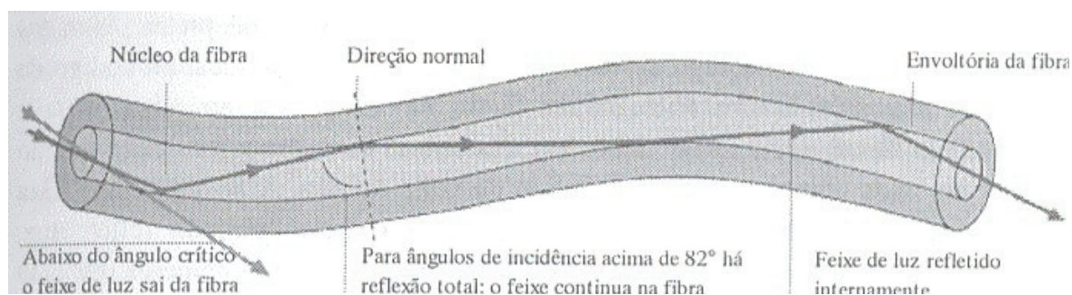
Fig. 9: Transmissão de luz através de uma fibra ótica.
