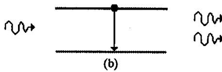
Fig.5b: emissão estimulada: “entra” um fóton e “saem” dois idênticos.
