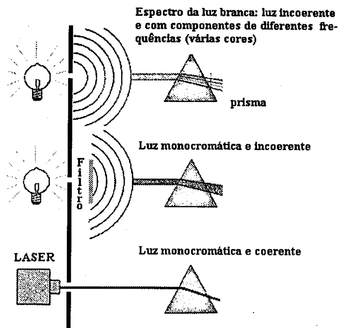
Fig. 7 – Comparação entre a luz de uma lâmpada de filamento e a do laser.
