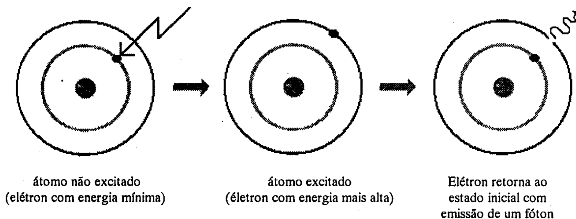
Fig. 4: Emissão de fótons por átomos excitados
