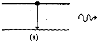
Fig.5a: emissão espontânea
